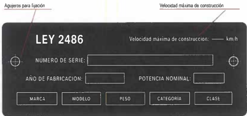
FIGURA 1. DISEÑO TÉCNICO DE LA LÁMINA DE MARCAJE PARA LEY 2486
